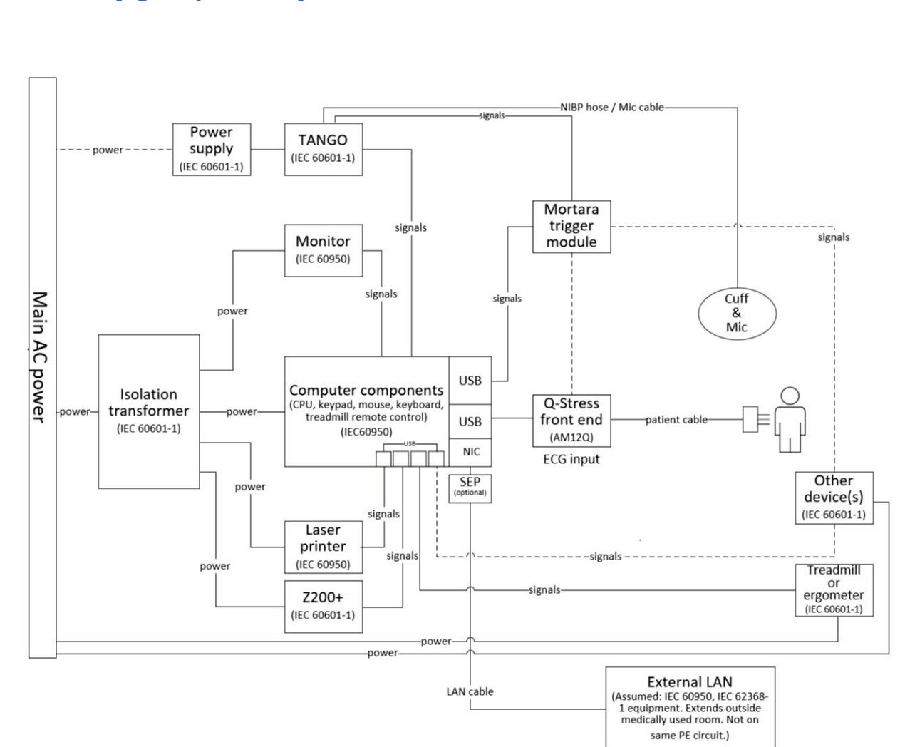
Slika 2 Dijagram povezivanja sustava Q-Stress
